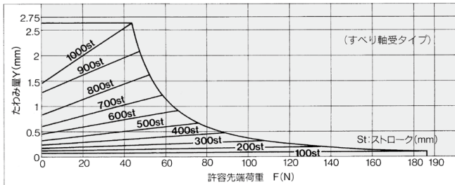
MGCM□50-ストローク-R
