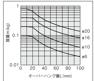
グラフ⑪ 負荷偏心量100mm
