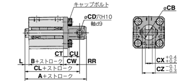
2山クレビス形
