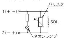
サージ電圧保護回路・ランプ付
