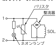
サージ電圧保護回路・ランプ付
