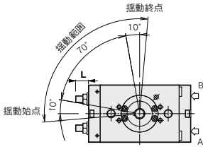
図は長軸側より見た場合
