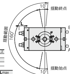
図は長軸側より見た場合
