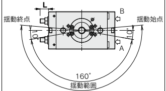
図は長軸側より見た場合
